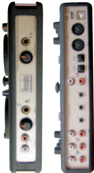
На задней части устройства наличествуют открытые оптические коннекторы
